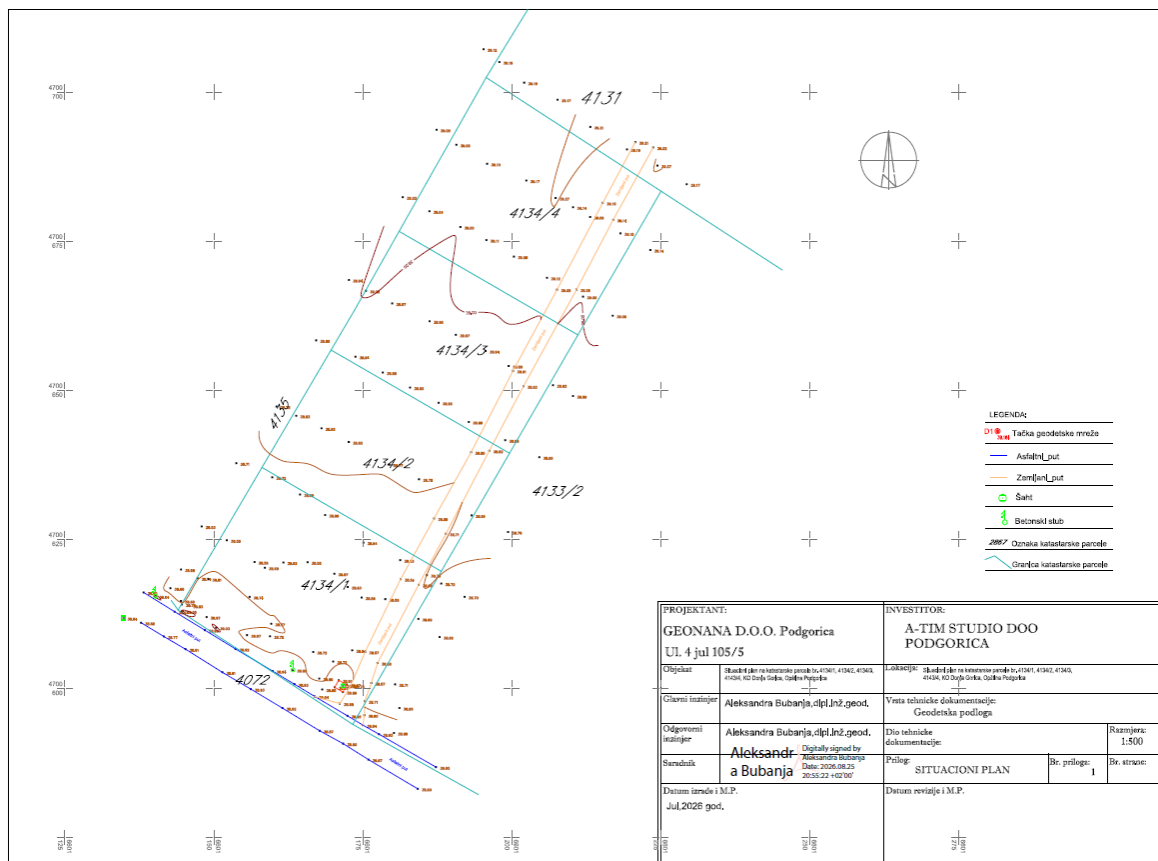
Slika 3: Zvanična geodetska podloga postojećeg stanja lokacije za građenje
