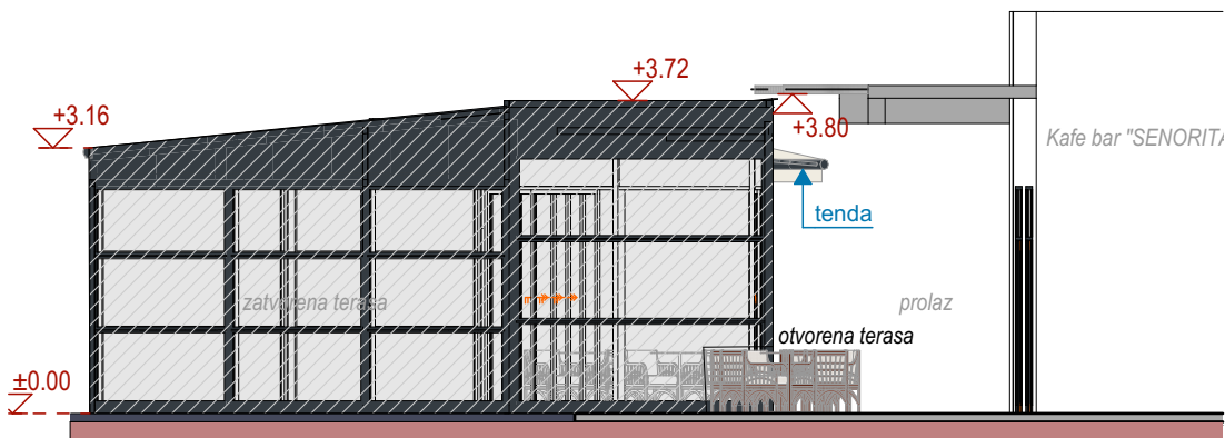
FASADA D-D
