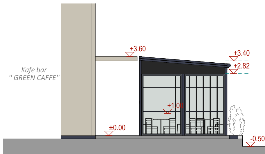
B Fasada 1:100
