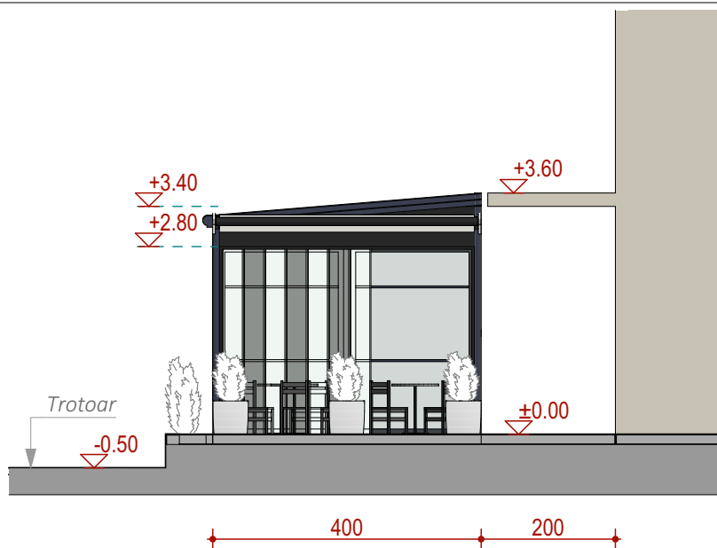
B Fasada 1:100
