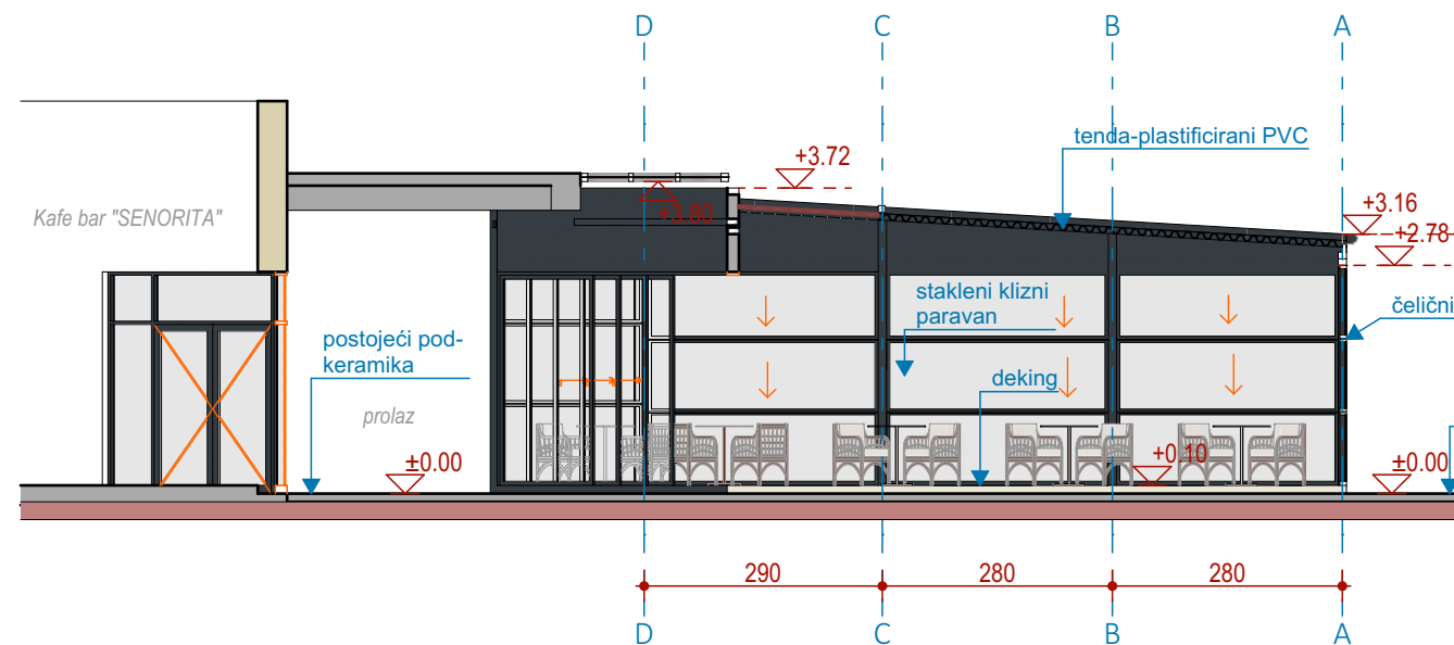
PRESJEK 3-3
