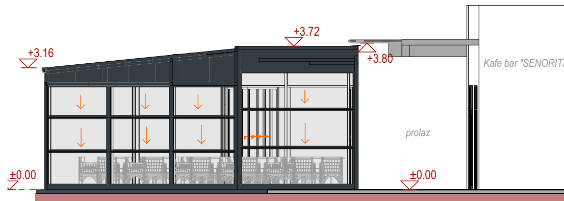
FASADA D-D
