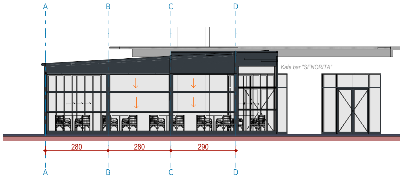
FASADA B-B
