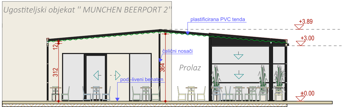
PRESJEK 1-1
