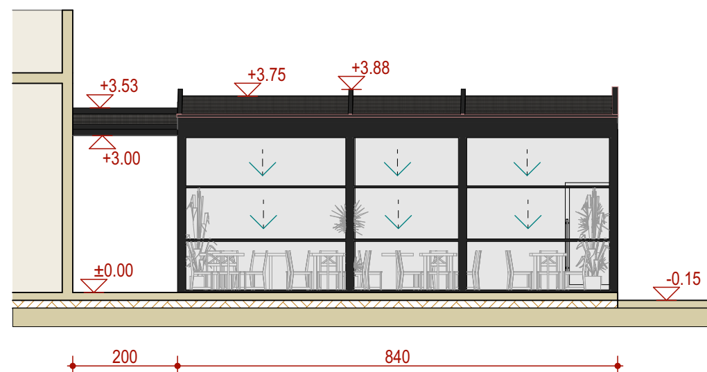
E-04 Elevation 1:100
