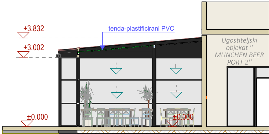
PRESJEK 3-3
