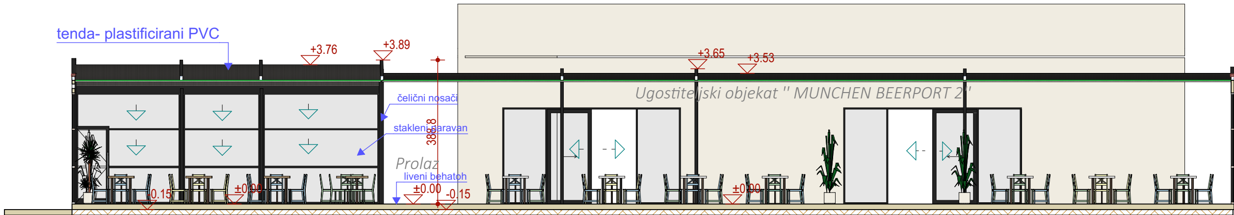
PRESJEK 2-2
