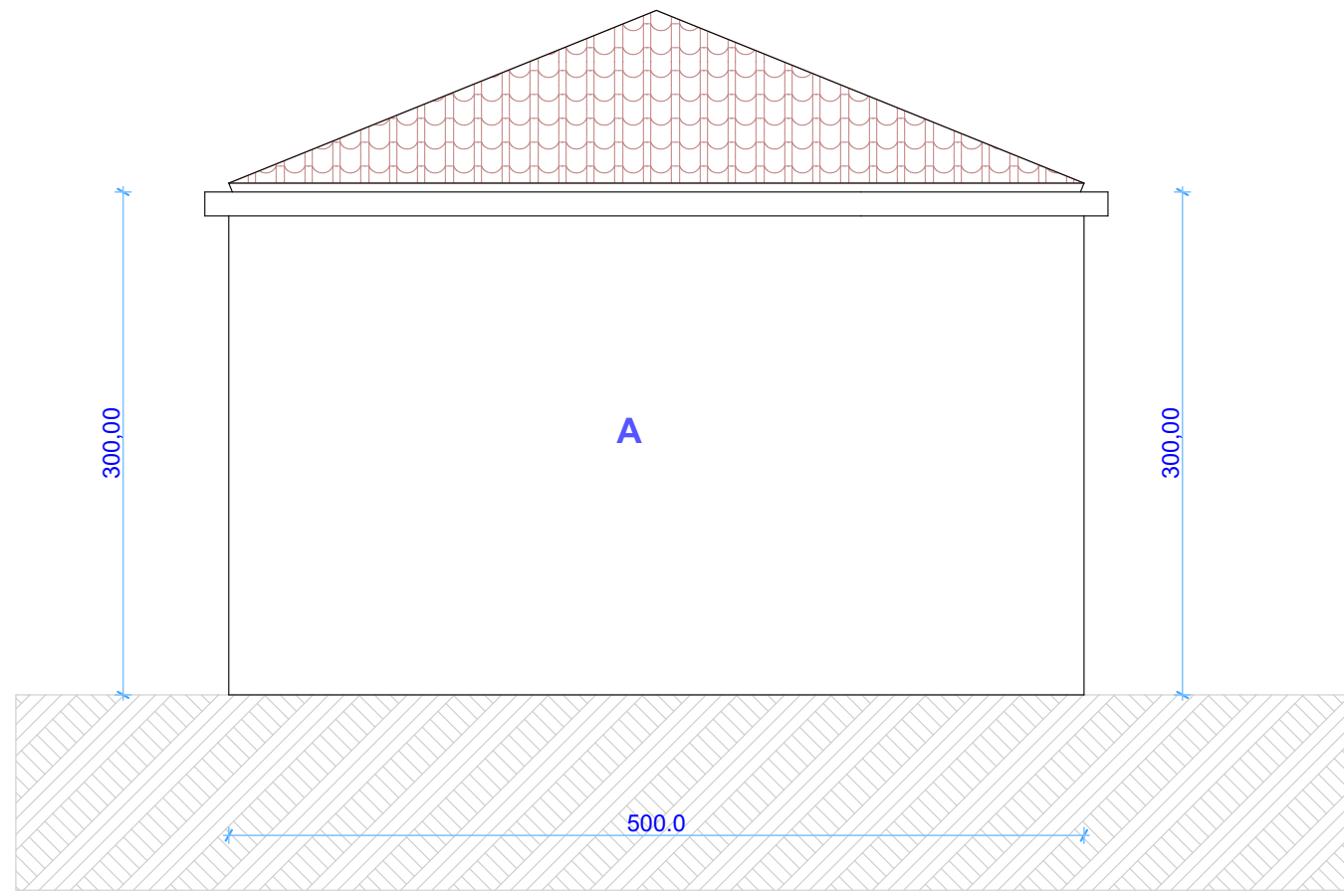
SJEVERNA FASADA
