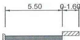
presjek 12-12
