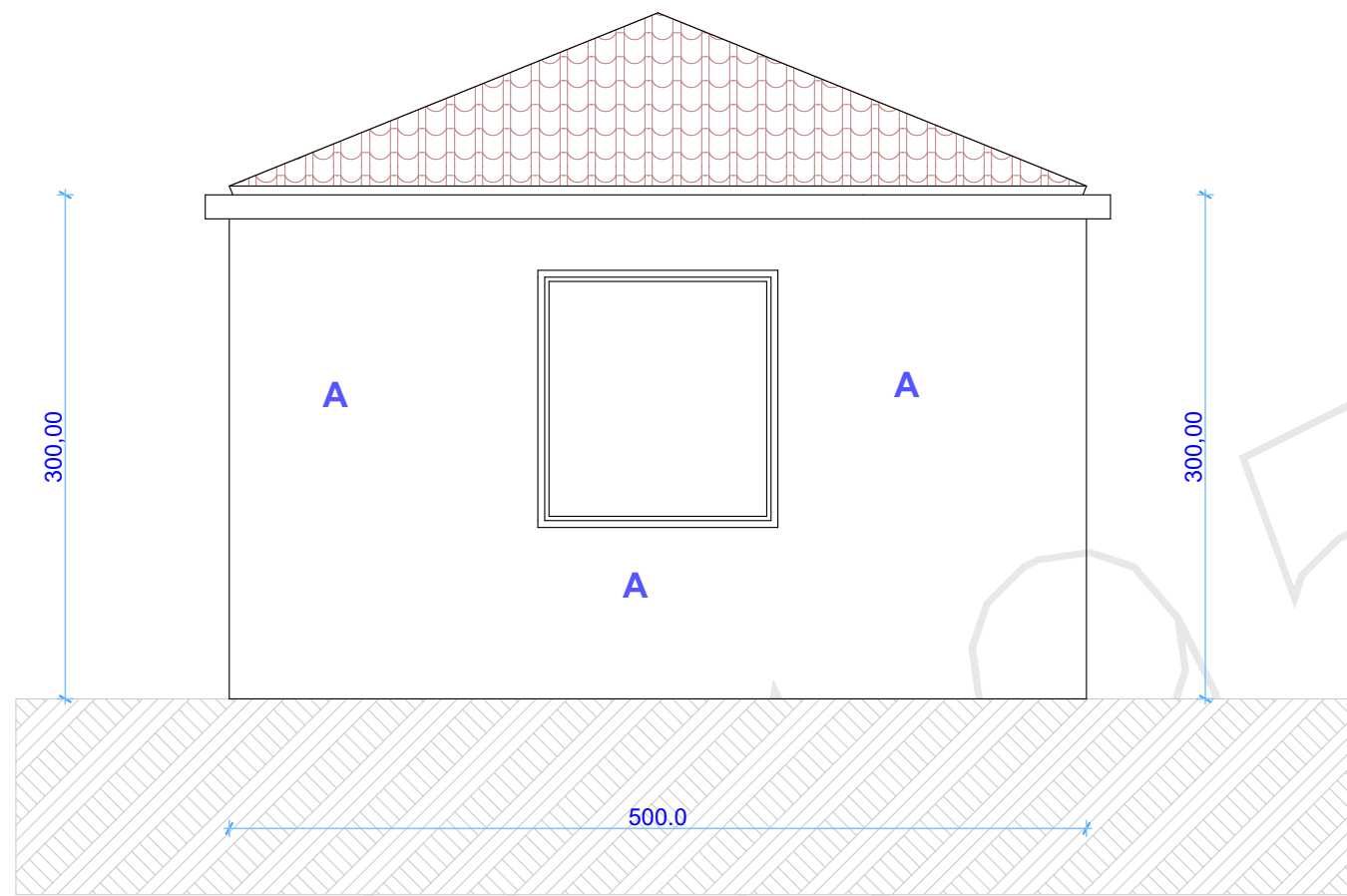
JUZNA FASADA
