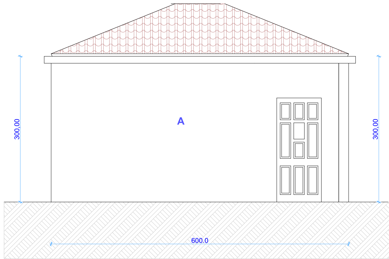
ZAPADNA FASADA
