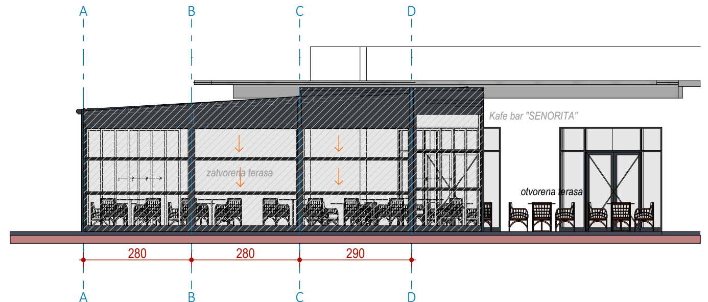
FASADA B-B
