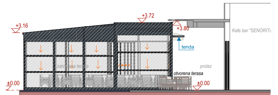
FASADA D-D
