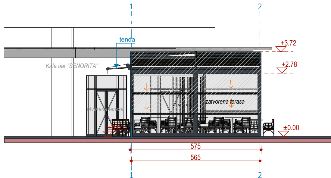
FASADA A-A
