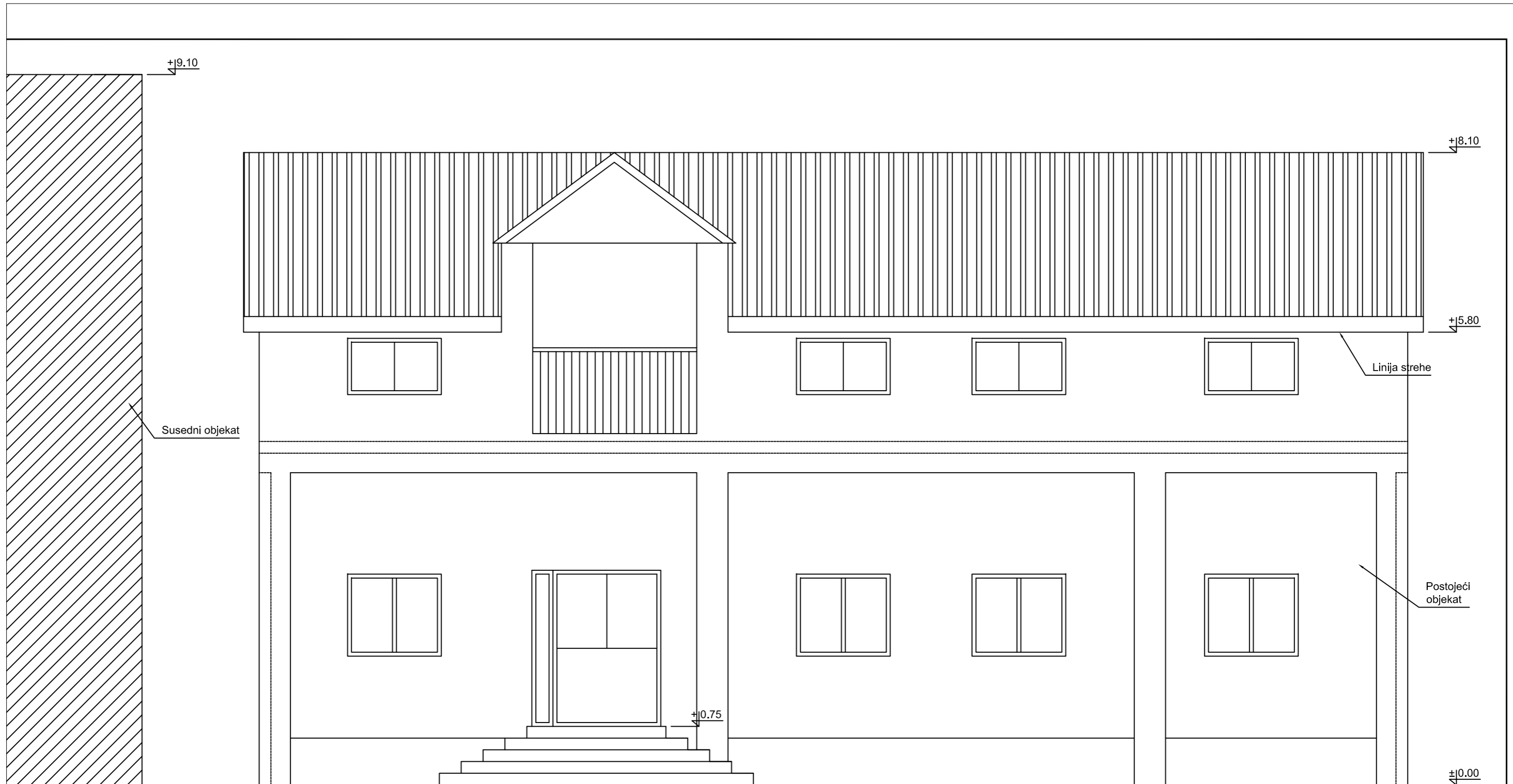
IZGLED 1-1 sa crteža IP.01
