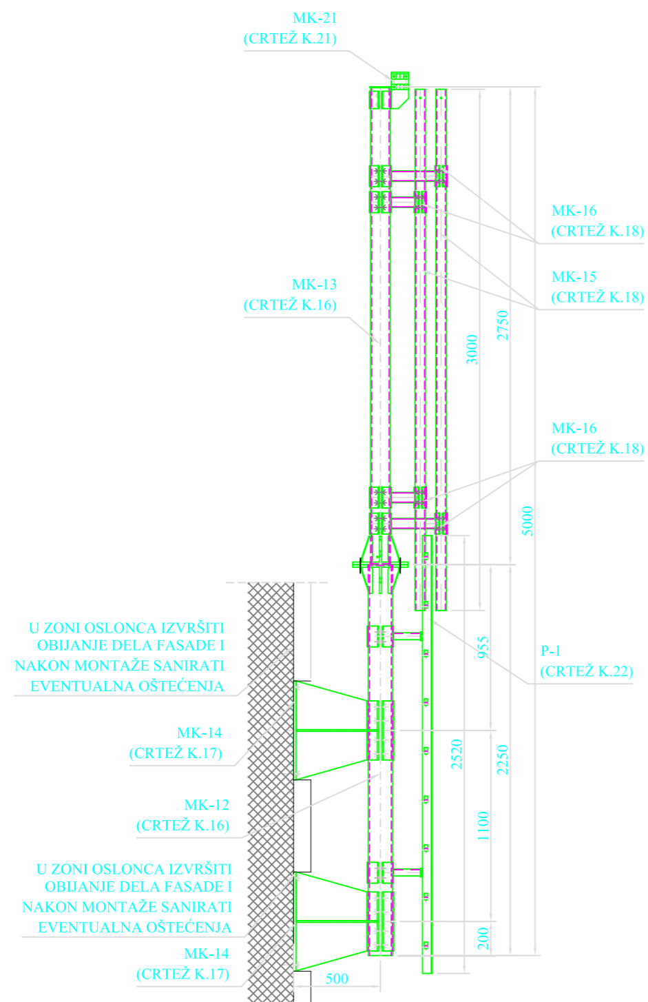
DISPOZICIJA NOSAČA ANTENA SEKTORA 1 I 2 - IZGLED
