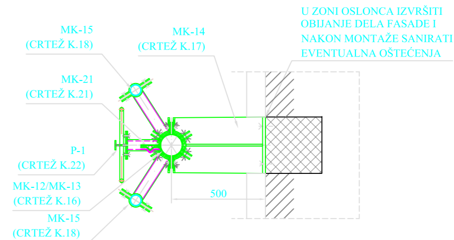
DISPOZICIJA NOSAČA ANTENA SEKTORA 1 I 2 - OSNOVA
