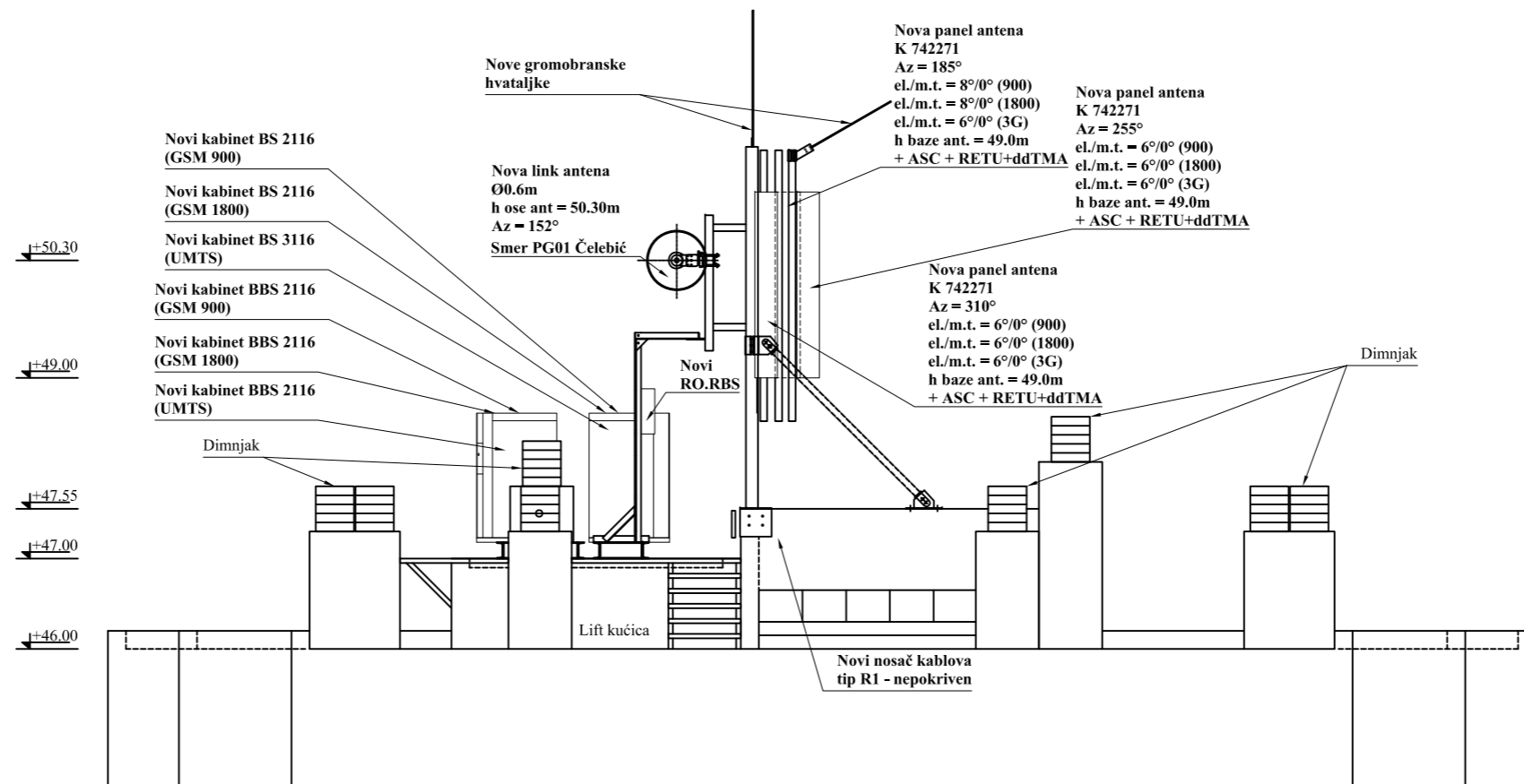
Izgleđ A-A sa crteža AG.04
