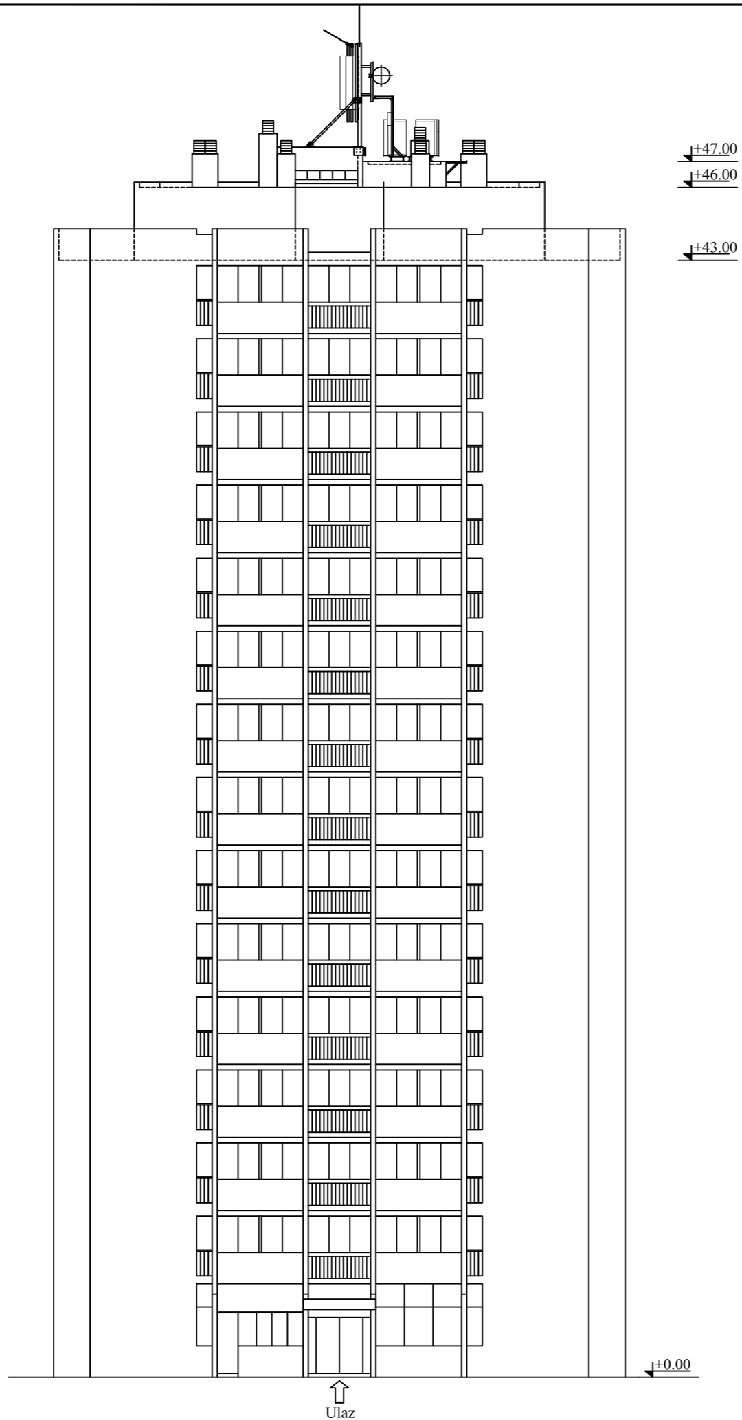
Izgled A-A sa crteža AG.04
