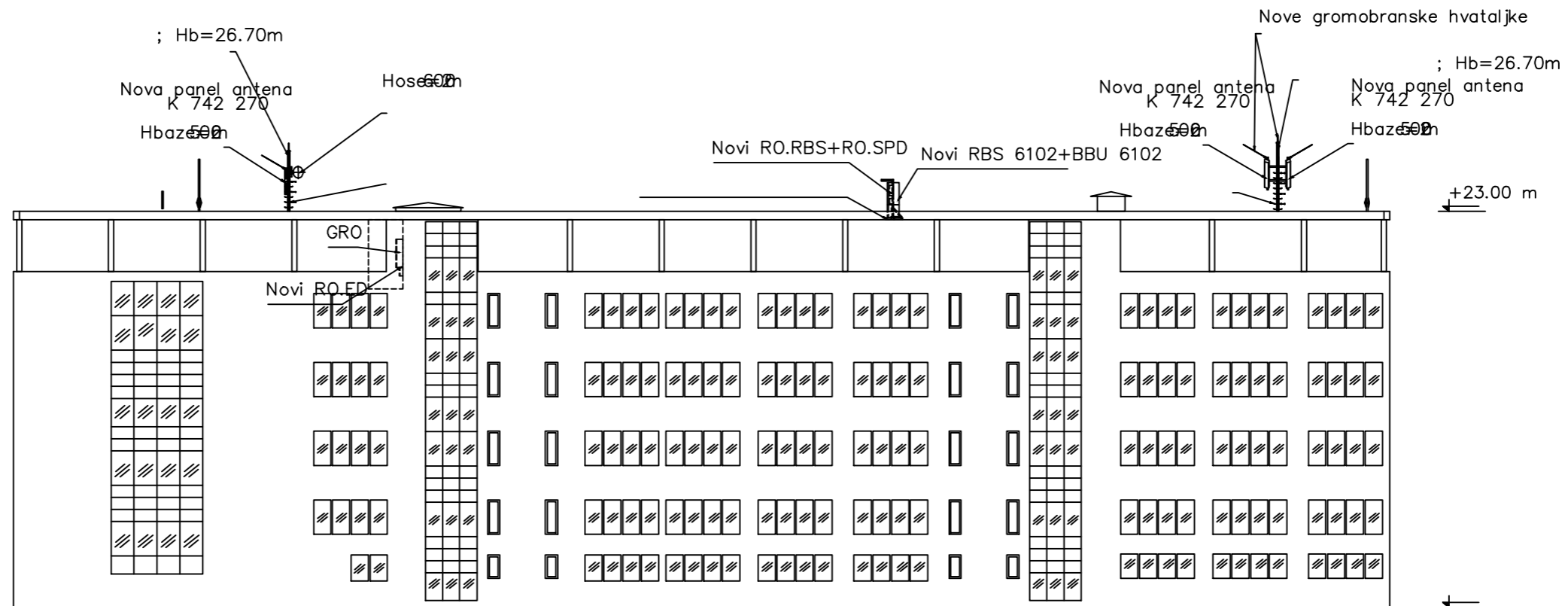
Izgled 2-2
