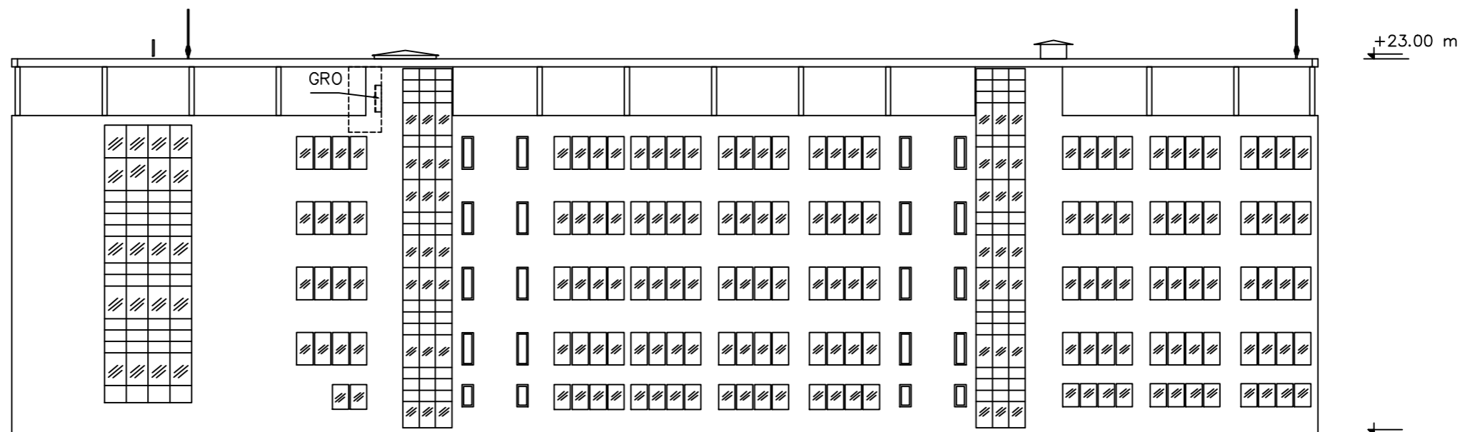
Izgled 1-1
