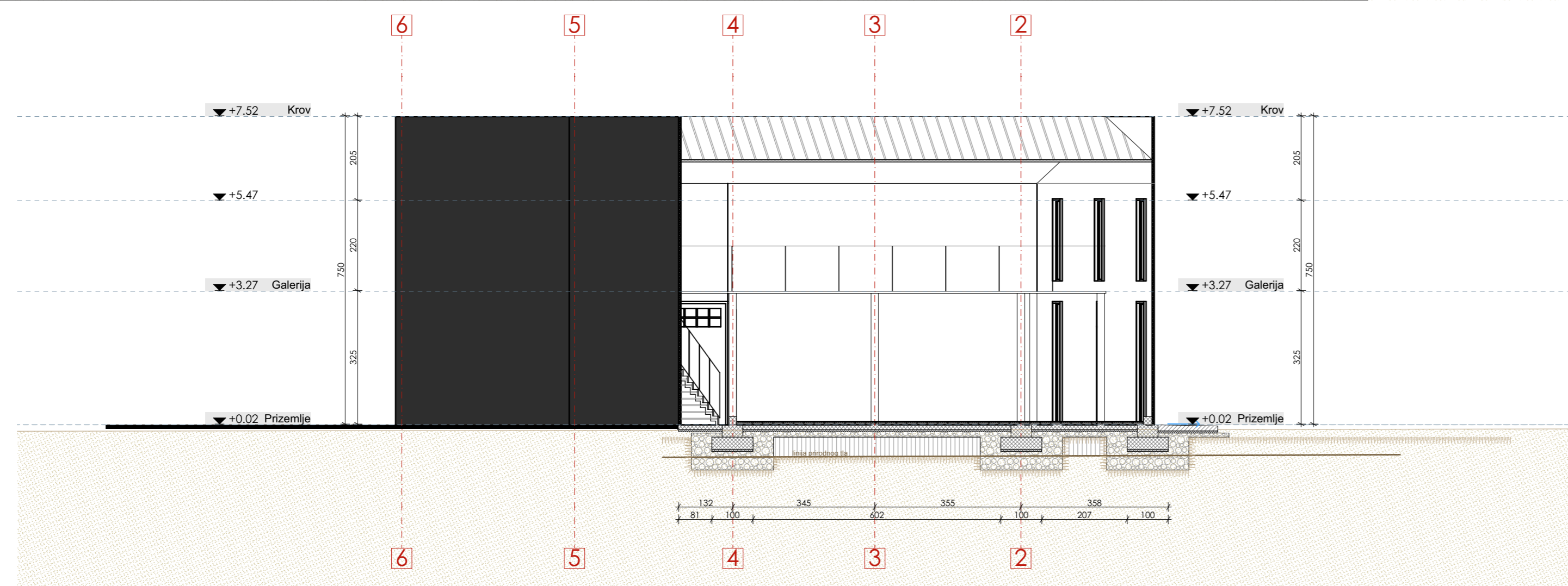
PRESJEK B - B
