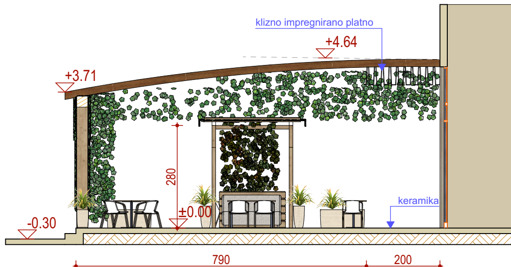
PRESJEK 2-2
