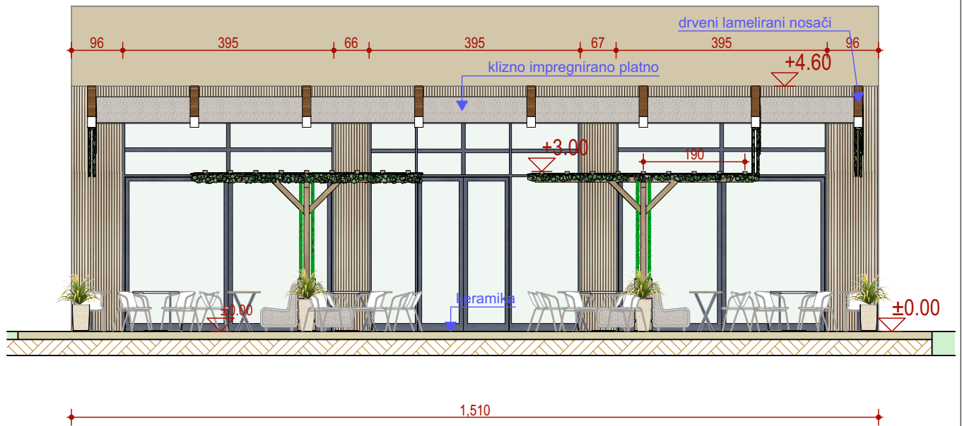
PRESJEK 1-1
