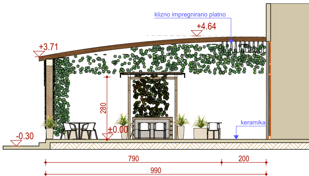
PRESJEK 3-3
