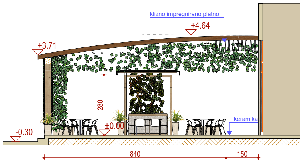
PRESJEK 3-3
