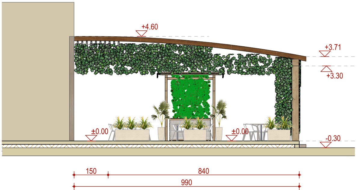
FASADA E-03
