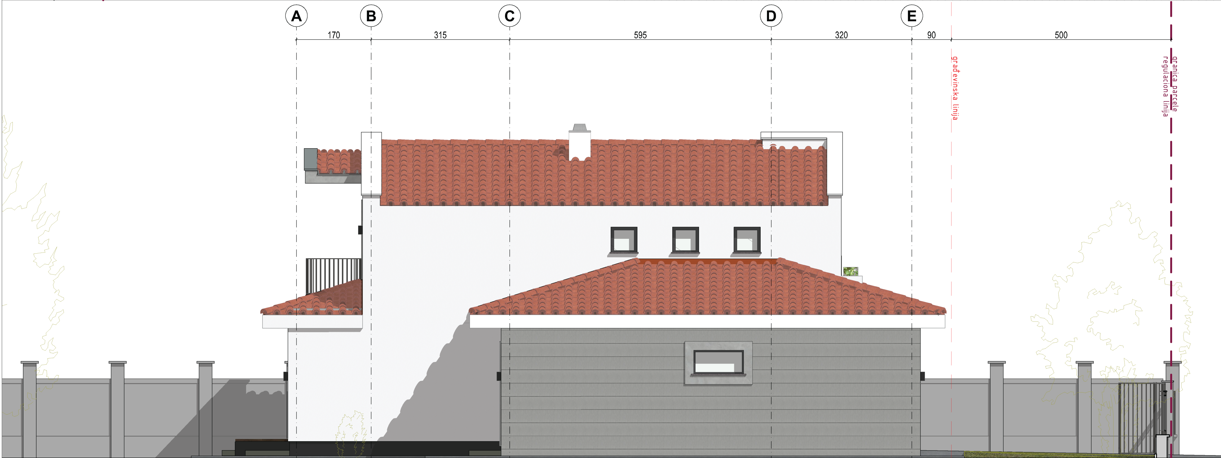
ZAPADNA FASADA
