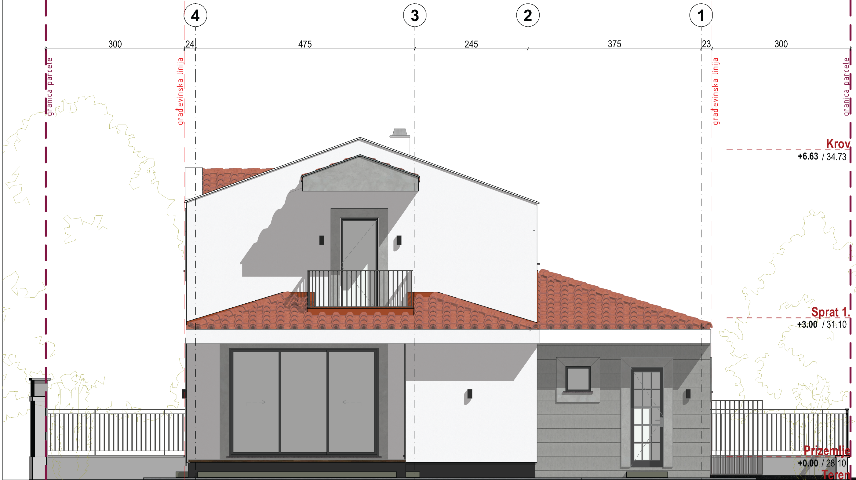
SJEVERNA FASADA
