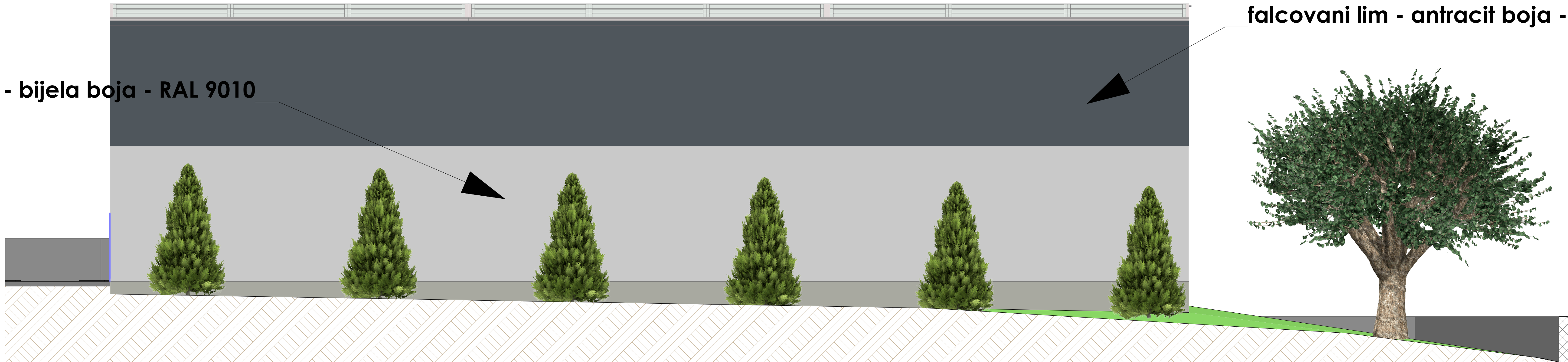
sjeveroistočna fasada
