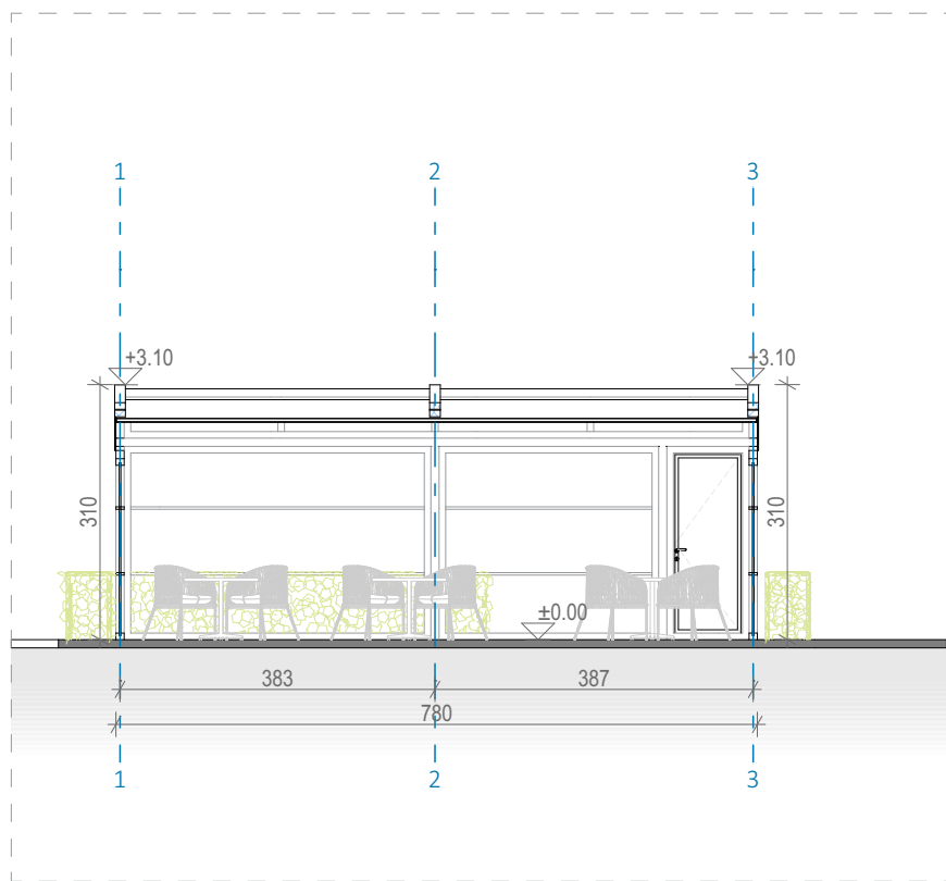
2 Presjek 2-2 1:100
