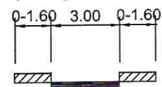
presjek 12-12
