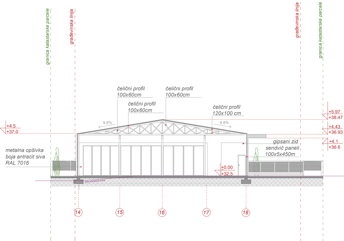
presjek 3-3
