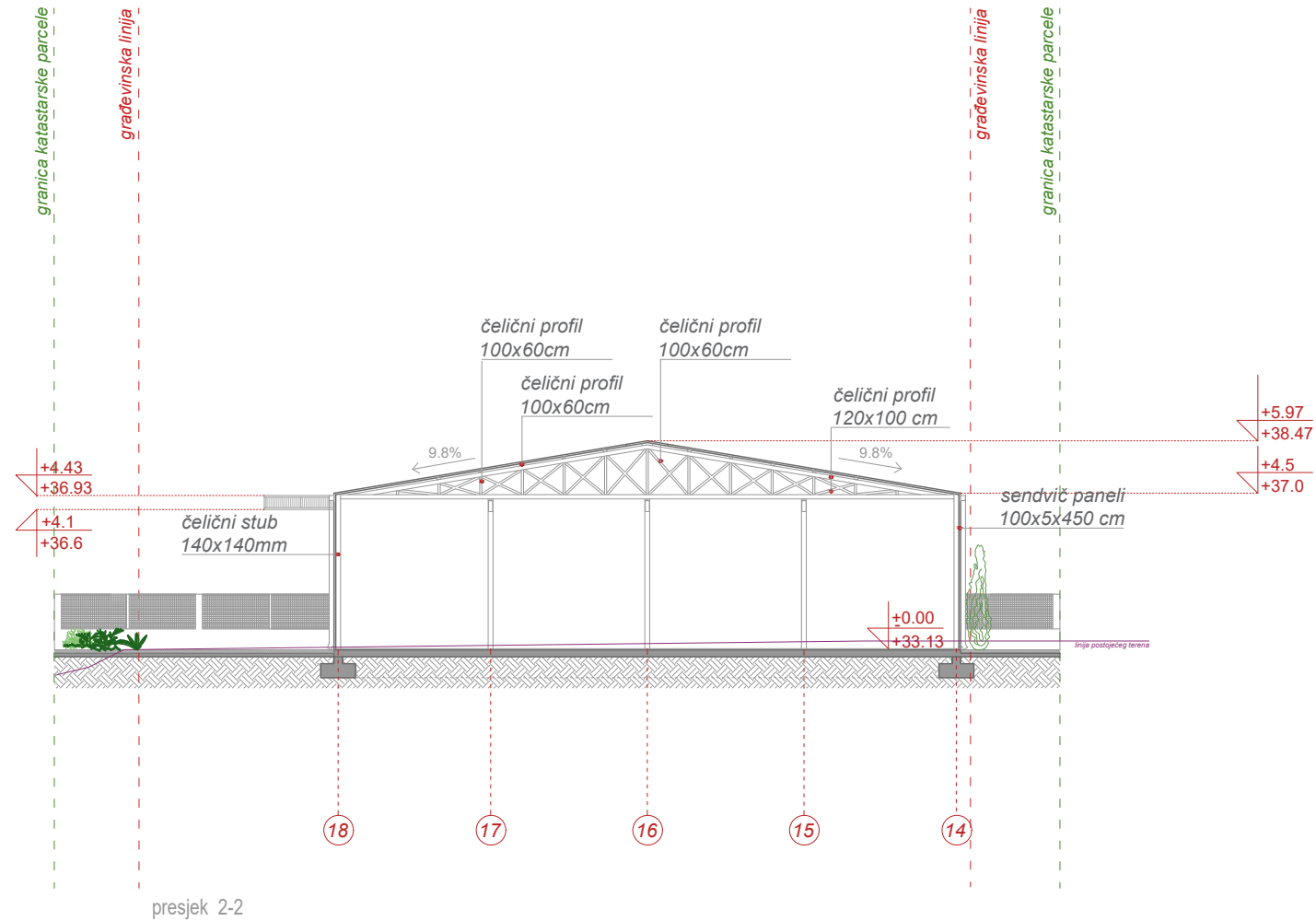
presjek 2-2
