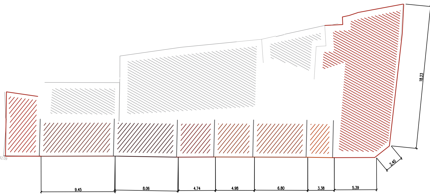
IZGLEDI FASADA SJEVERNOG FRONTA
