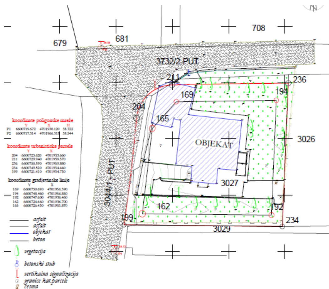
Slika 3: Zvanična geodetska podloga postojećeg stanja lokacije za građenje
