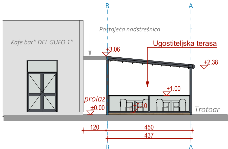
C Elevation 1:100
