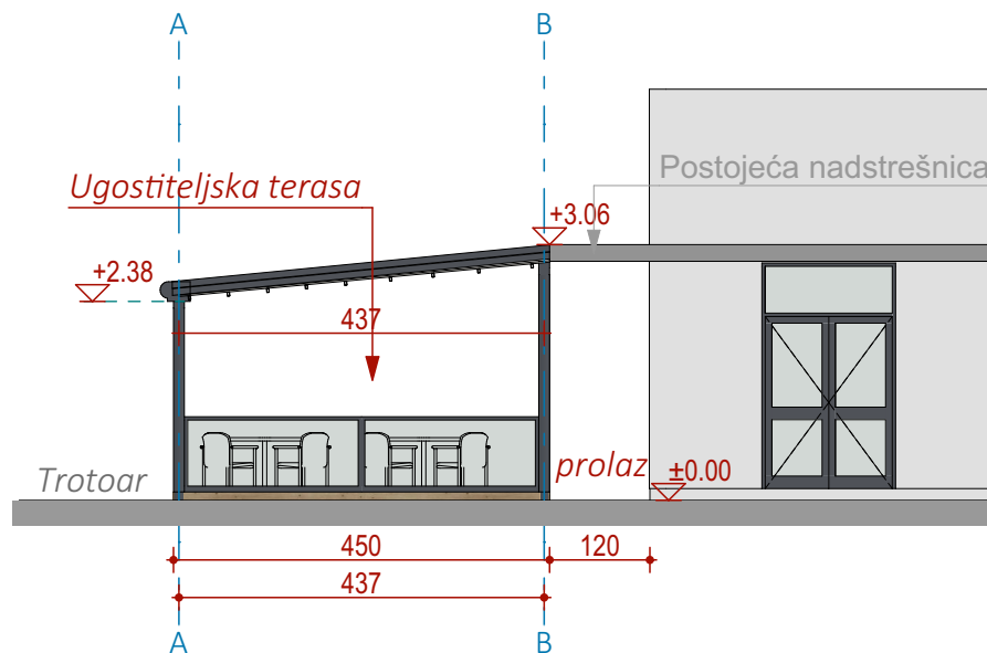
B Elevation 1:100
