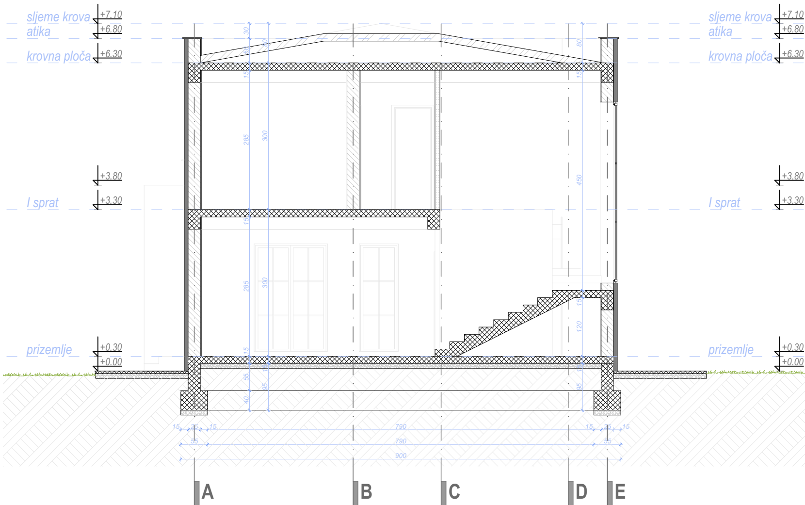
presjek 1-1
