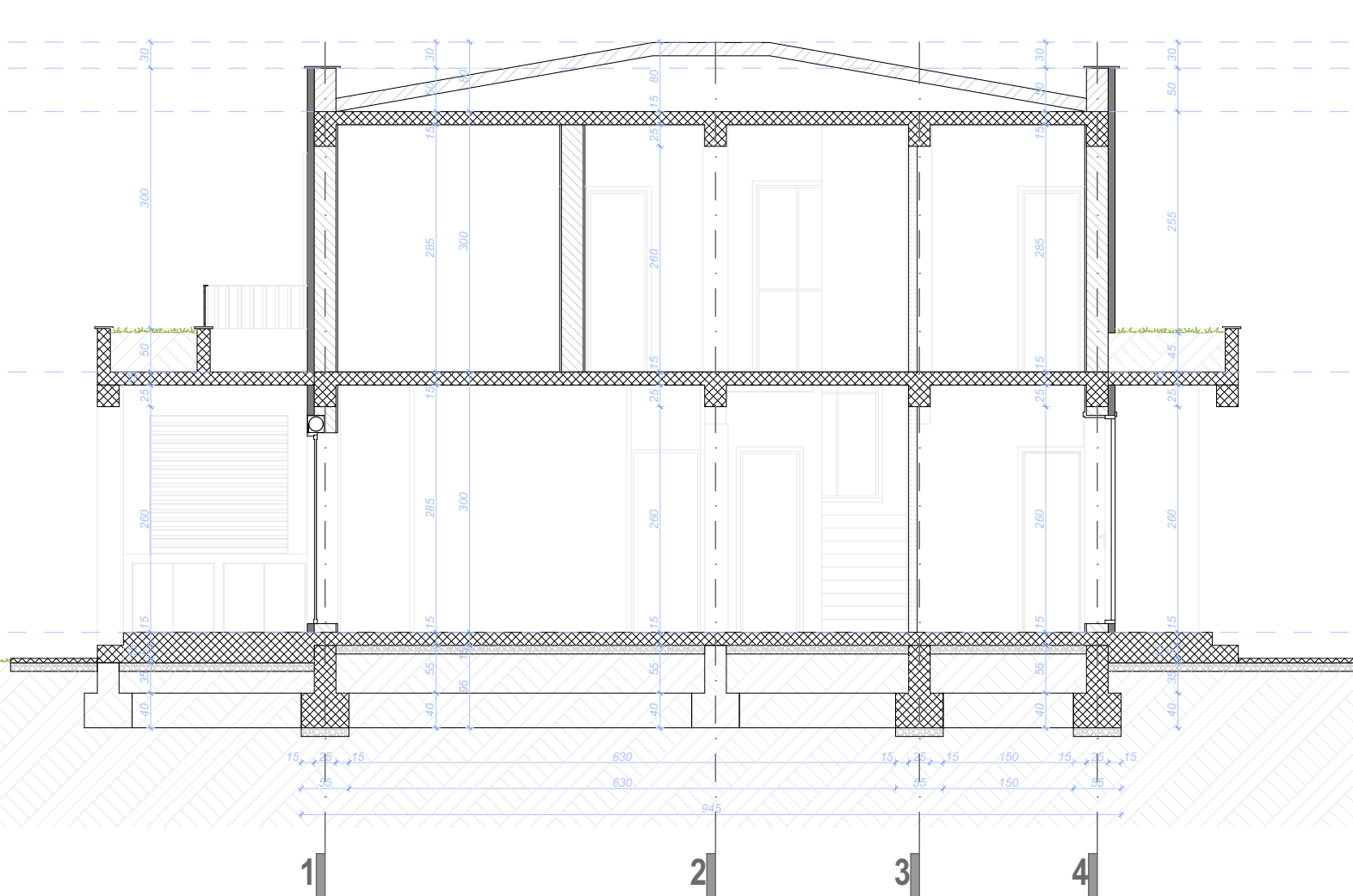
presjek 2-2
