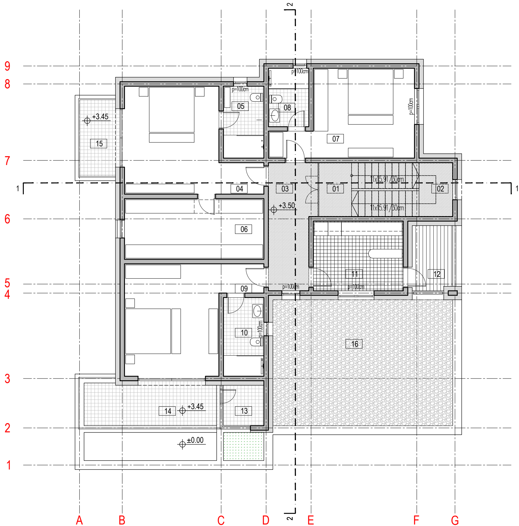
LEGENDA MATERIJALA, OZNAKA I NAMJENE POVRŠINA
