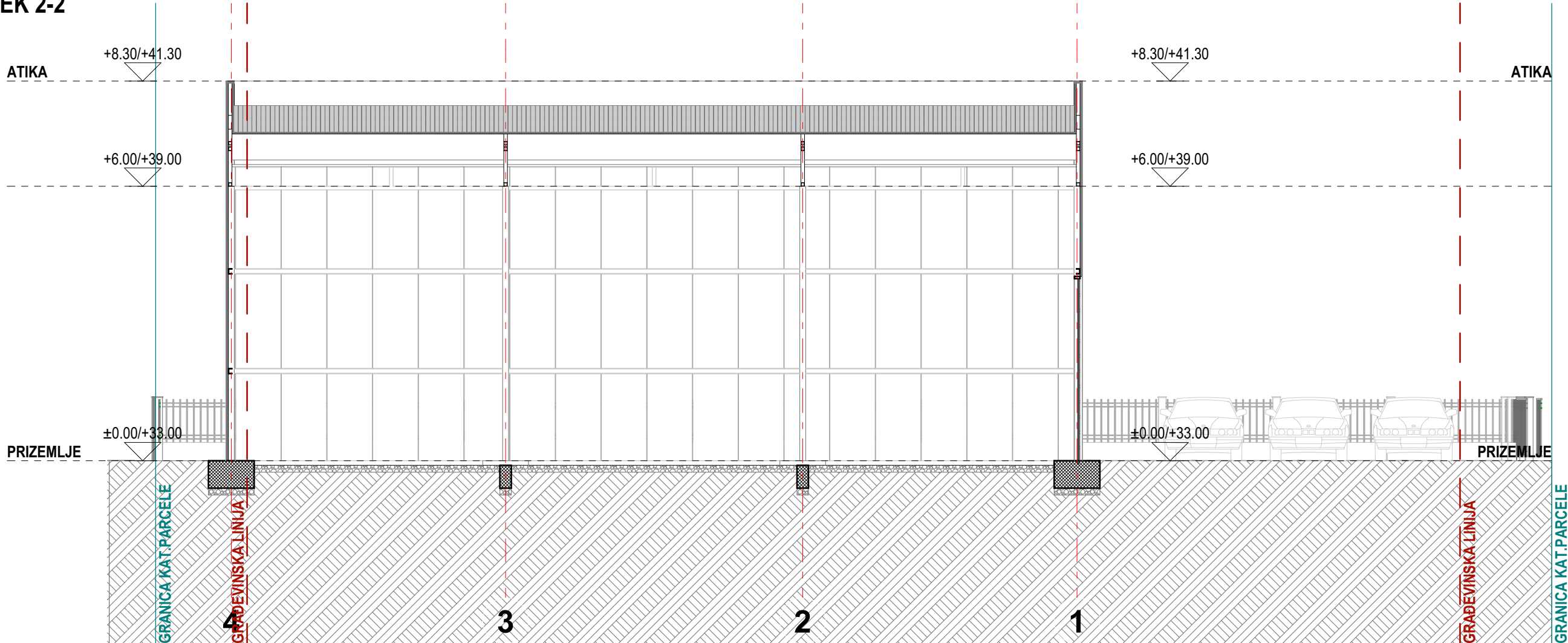
PRESJEK 2-2
