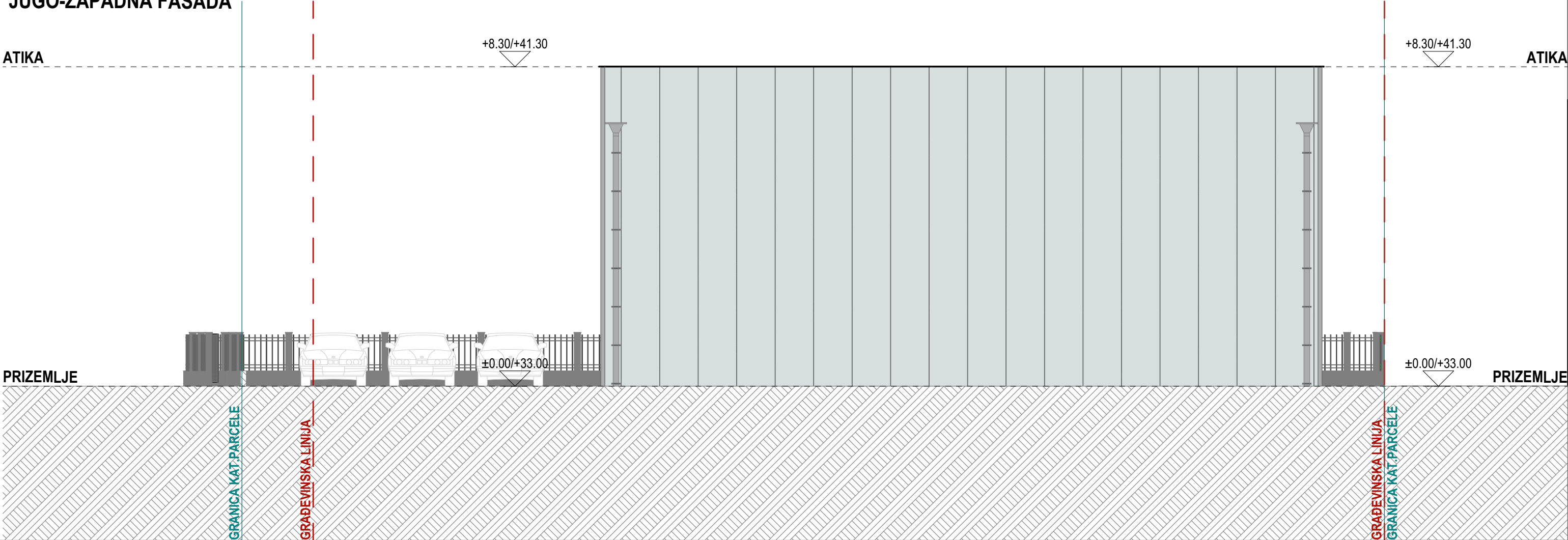
JUGO-ZAPADNA FASADA
