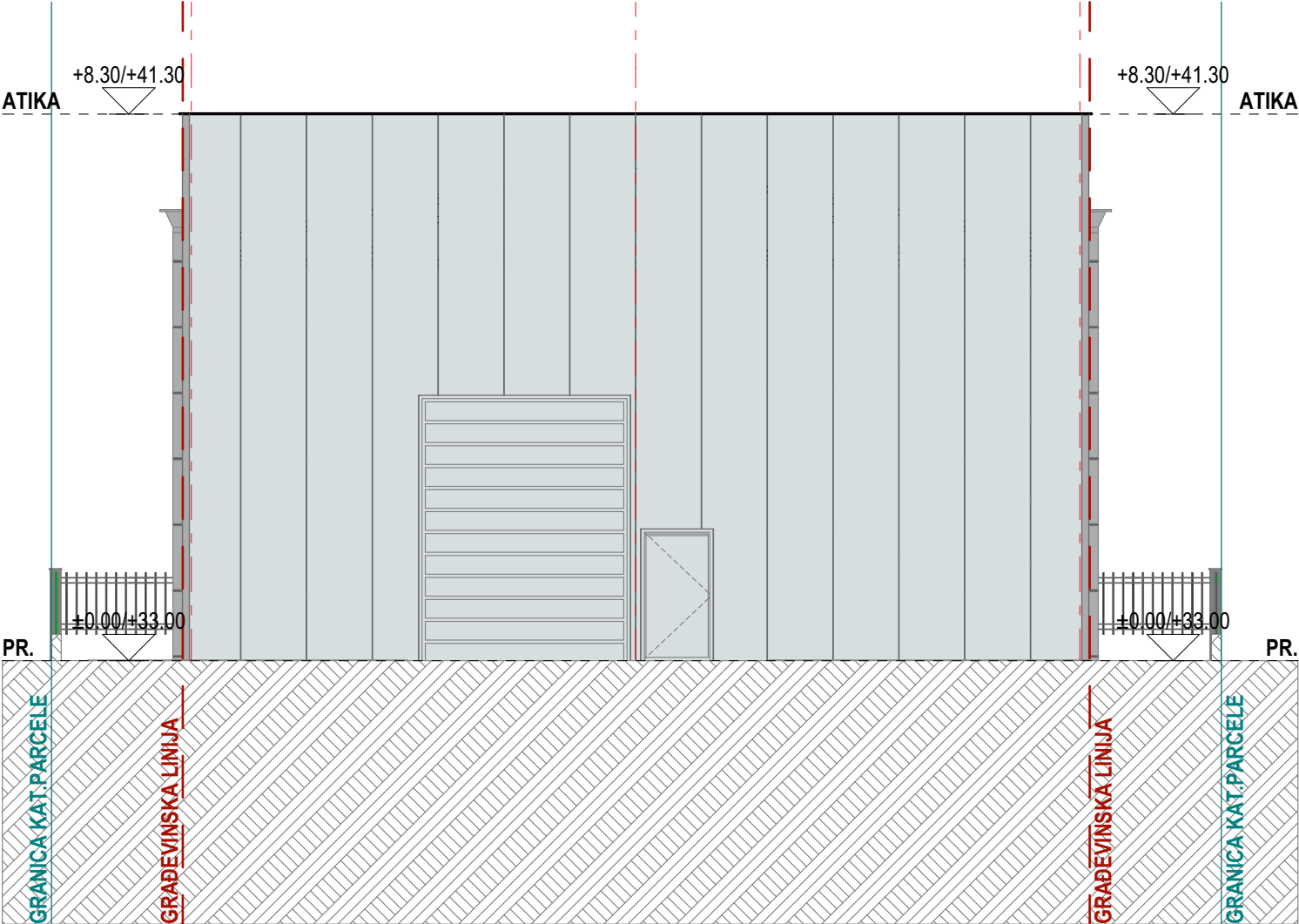
SJEVERO-ZAPADNA FASADA
